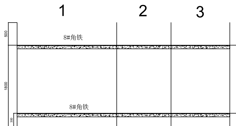
装置5-5剖面图&填料支架安装图
