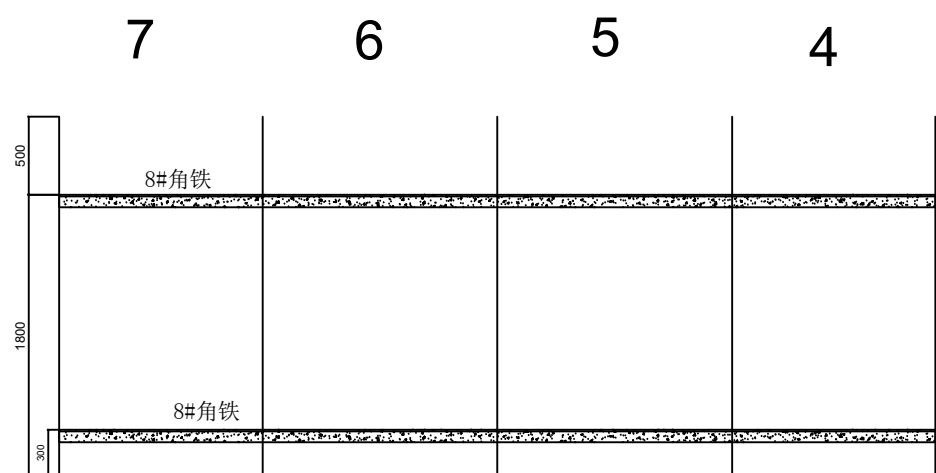
装置6-6剖面图&填料支架安装图
